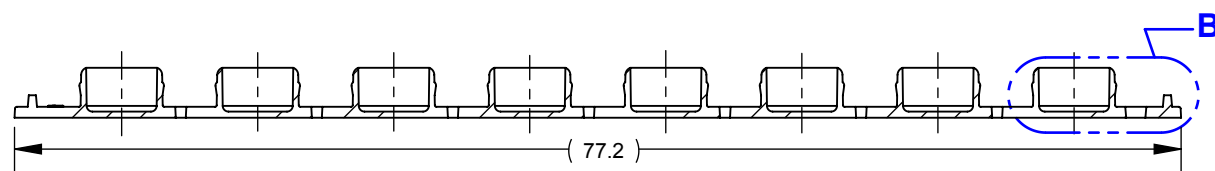
SECTION A-A SCALE 2 : 1
